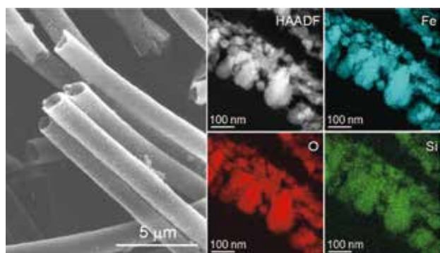
鉄酸化細菌が形成したチューブ状酸化鉄とその微細構造 Tubular iron oxides of bacterial origin and their nanostructures
