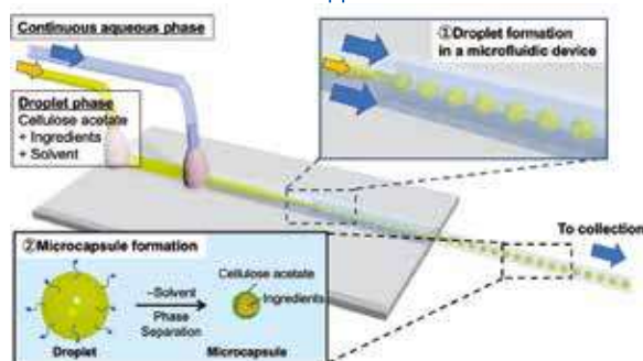
図1：マイクロ流路を用いたフロープロセスによる酢酸セルロースマイクロカプセルの調製
